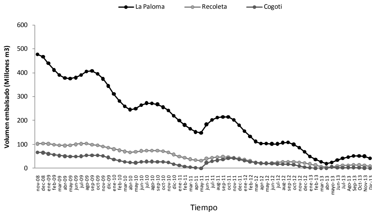
Figura E2. Evolución de los embalses de la provincia de Limarí para el periodo 2008 – 2013
