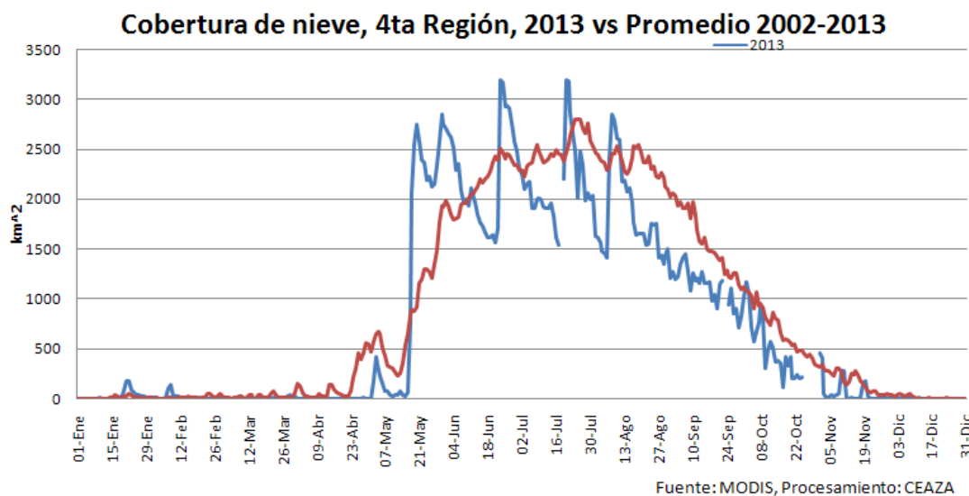
Figura 15. Cobertura de nieve año 2013 contrastado con valor histórico período 2002 – 2013 de la Región de Coquimbo.
