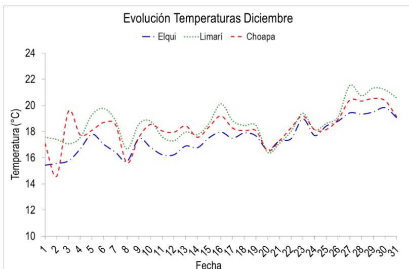
Figura 5. Promedios de temperatura superficial diaria en diciembre de 2013 obtenidos a partir de estaciones CEAZA-Met.
