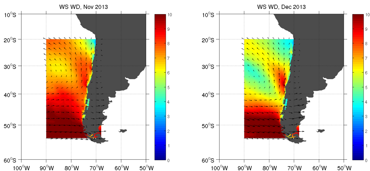
Figura 4. Velocidad y dirección de los flujos de viento (m/s) promedio predominantes en noviembre y diciembre, datos re-análisis NCEP/FNL.
