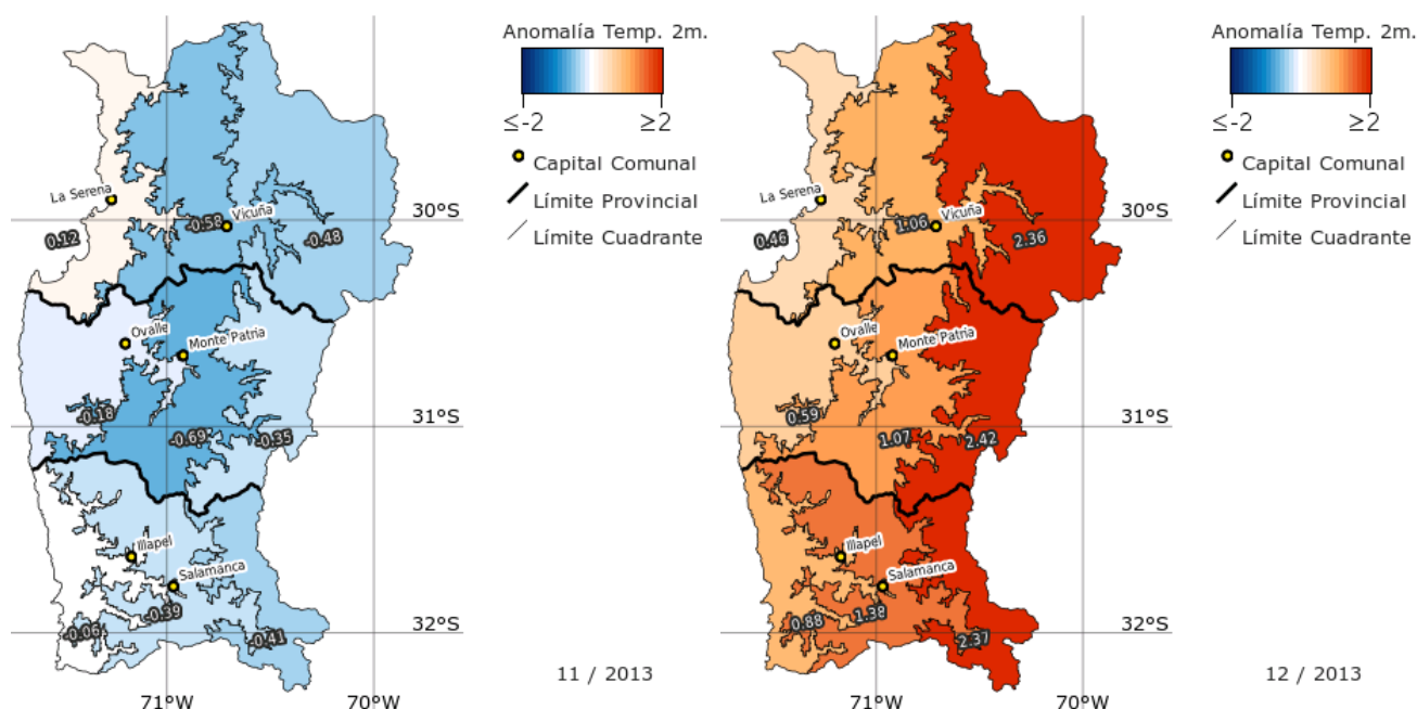
Figura 7. Anomalías de temperatura superficial promedio en noviembre (izquierda) y diciembre (derecha), modelo WRF CEAZA
