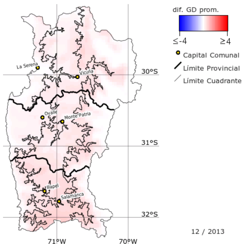
Figura 9b. Mapa de diferencias de Grados Día entre diciembre 2012 y diciembre 2013 (fuente: simulación WRF CEAZA)
