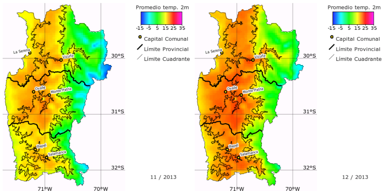
Figura 6. Promedios de temperatura superficial en noviembre (izquierda) y diciembre (derecha), modelo WRF CEAZA.
