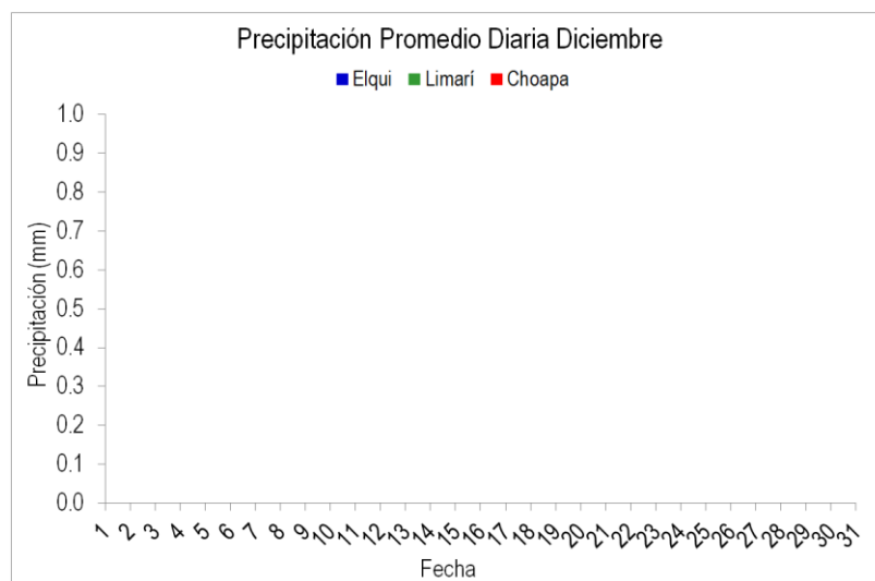
Figura 10. Precipitaciones en las tres provincias de la Región de Coquimbo, CEAZA-Met, diciembre 2013.
