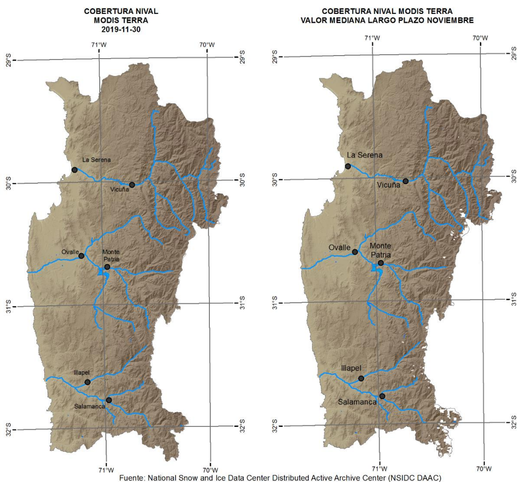
Figura N1. Mapa de la cobertura de nieve el último día del mes actual (izquierda) y el mapa con las medianas del mes de período 2002-2018 (derecha)
