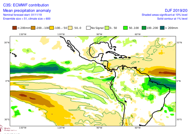
Figura PE1. Pronóstico de las anomalías de precipitación para el próximo trimestre (fuente: C3S).
