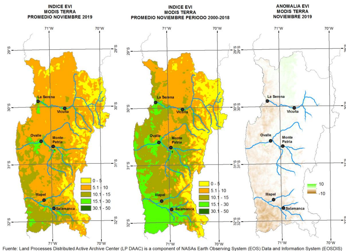
Figura EVI 1. Mapa promedio del EVI del último mes en la Región de Coquimbo (izquierda). Mapa promedio climatológico del período 2000-2018 (centro). Mapa de la anomalía mensual (derecha).
