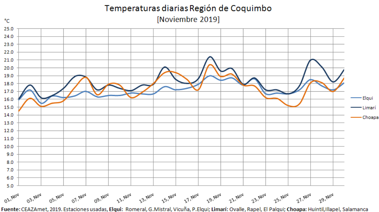
Figura VT1. Promedios diarios de temperatura [ ^{\circ}\text{C} ] a 2 m en el mes pasado obtenidos a partir de la red CEAZA-Met [www.ceazamet.cl].
