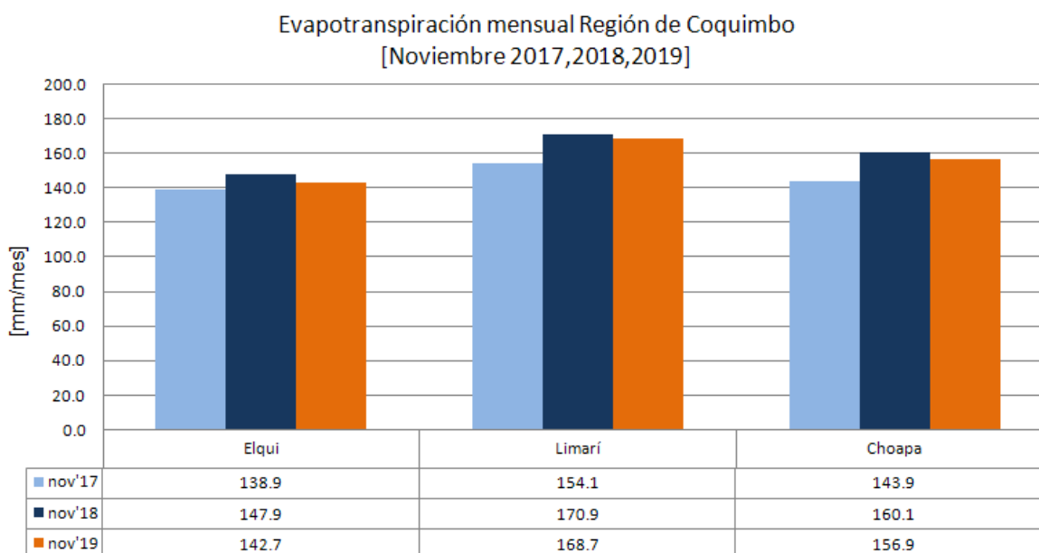
Figura Et1 y Et2. Evolución de la evapotranspiración para los últimos 12 meses (arriba) y comparativa con igual mes de los años 2017 y 2018 (abajo), obtenida a partir de estaciones CEAZA-Met.
