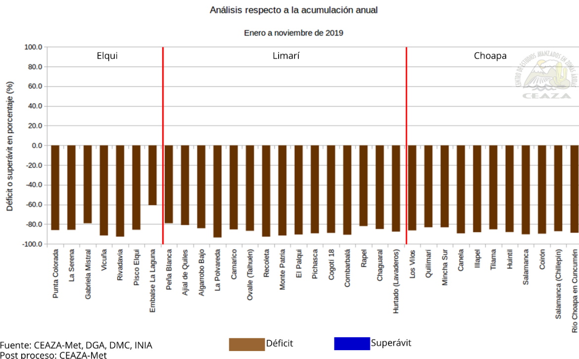
Figura P2. Análisis porcentual de las precipitaciones acumuladas durante el año 2019. Período base climatológico: 1981-2010. Fuente: CEAZA-Met, DGA, DMC e INIA.
